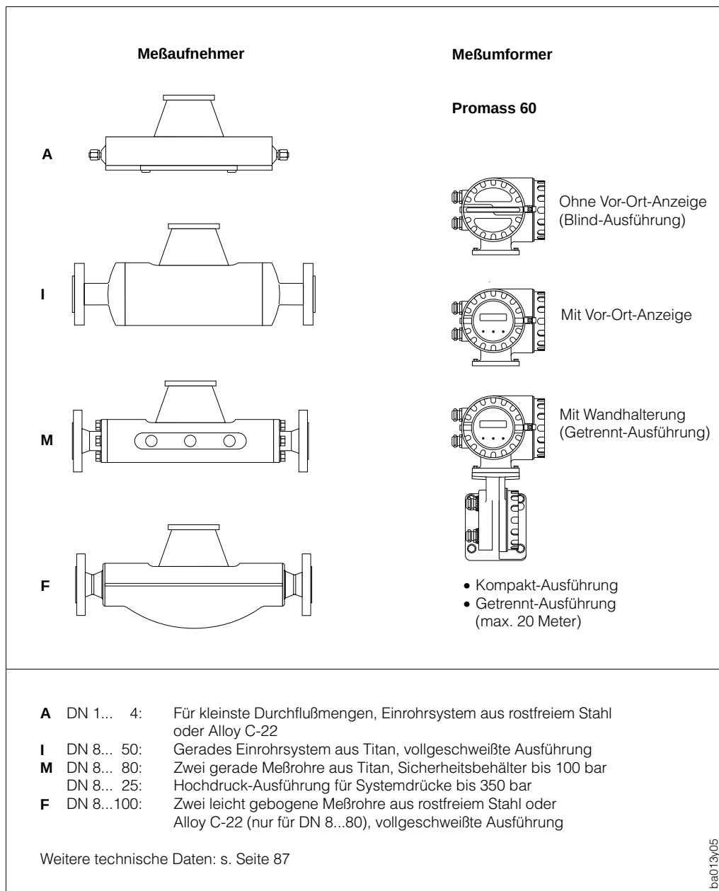
Abb. 3: Promass 60-Meßsystem
