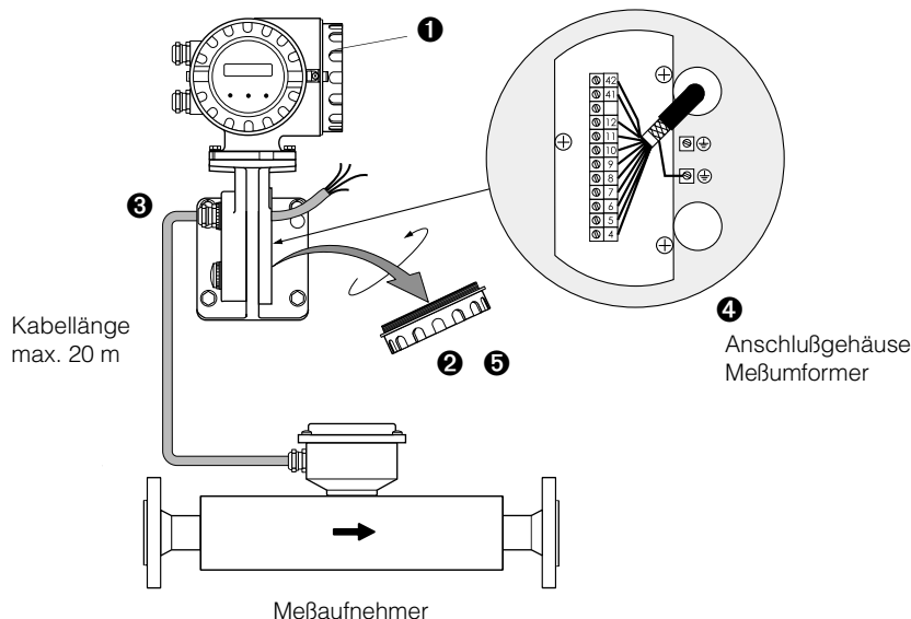
Anschlußgehäuse Meßumformer
